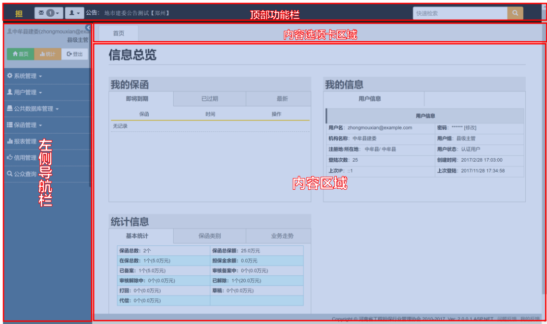
图 0.3-2 登陆后首页界面
